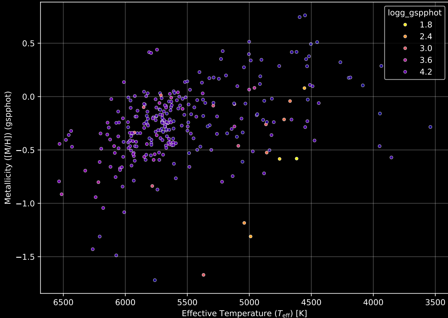
GALAH DR4 Field: [6954] Stellar Population Parameters (n= 293)
