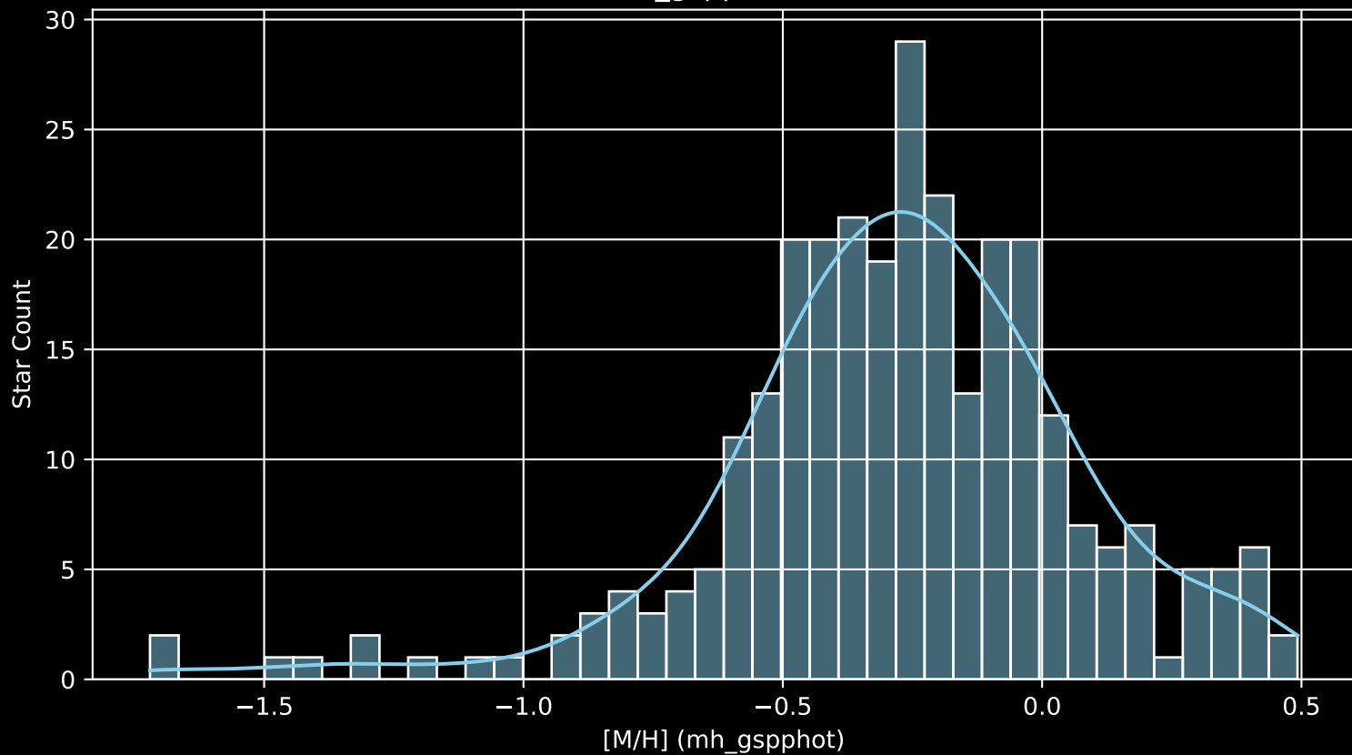
GALAH DR4 Field: [6954] [M/H] (mh_gspphot) (n= 289)
