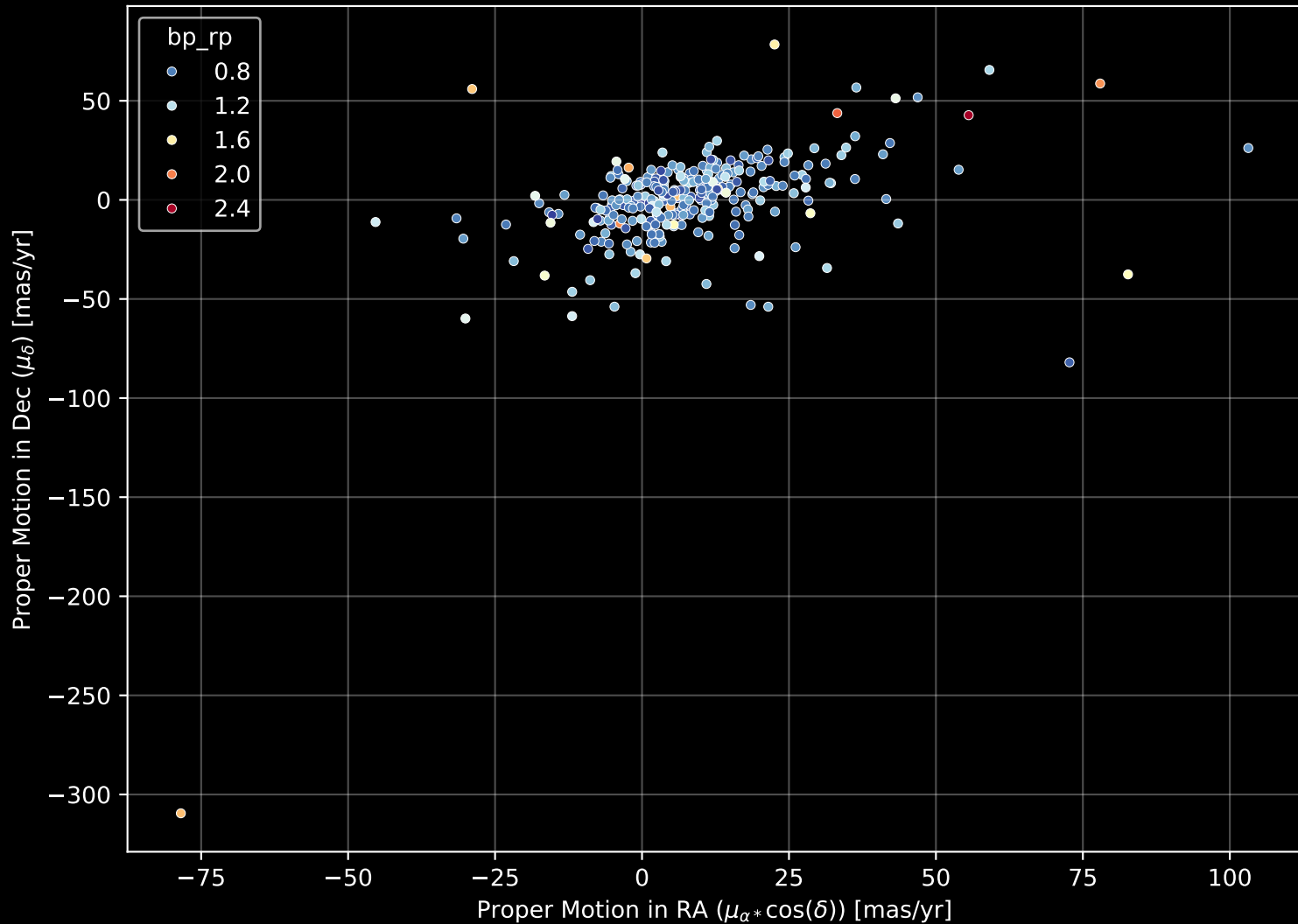
GALAH DR4 Field: [6954] Proper Motion Diagram (n= 293)
