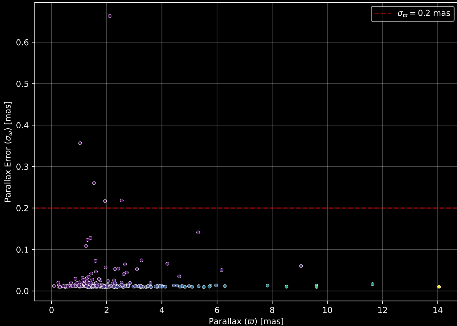
GALAH DR4 Field: [6954] Parallax Quality (n= 293)
